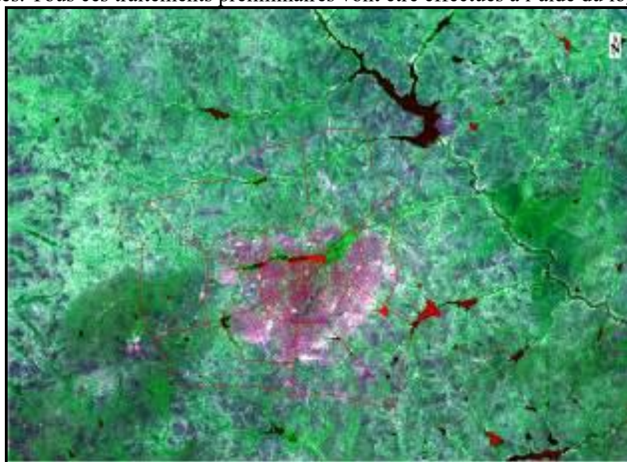
Figure 3. Composition colorée (MIR/PIR/R) (Source : Zabré N. G., Traitement des données)
