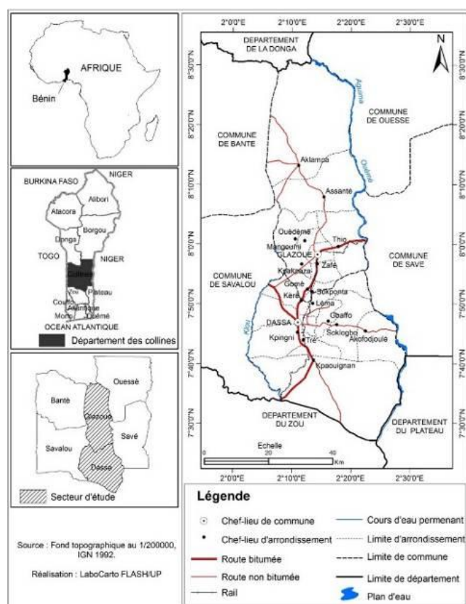
Figure 12: Situation géographique des Communes de Dassa-Zoumé et de Glazoué Source : Fond topographique au 1/200000, IGN 1992
