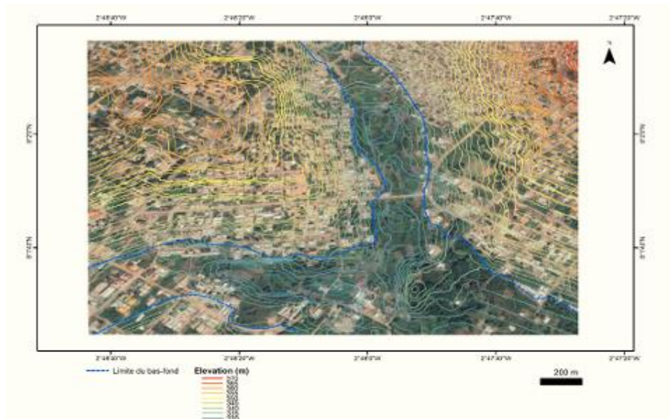
Figure 10 : Occupation du sol selon l'hypsométrie de la séquence spatiale de Bondoukou (Source : Google Earth, 2022 ; Réalisation : Bini K. E., 2024)
