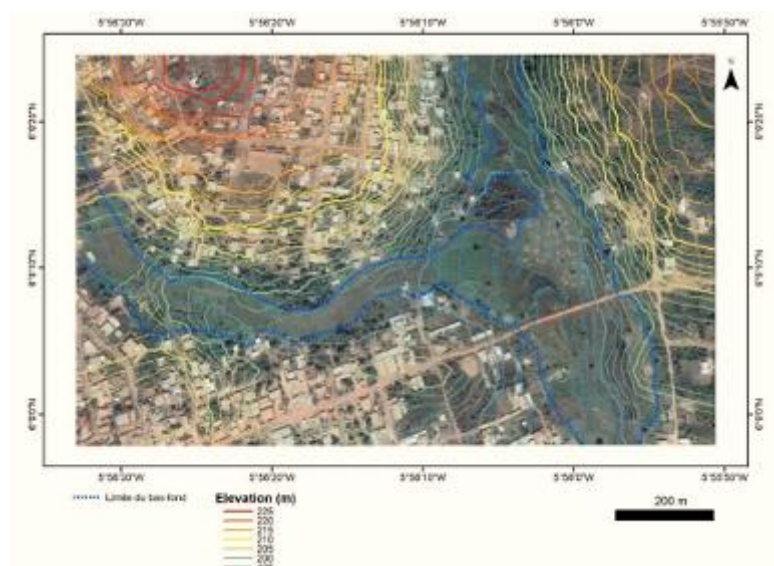
Figure 8 : Occupation du sol selon l'hypsométrie de la séquence spatiale de Gagnoa (Source : Google Earth, 2022 ; Réalisation : Bini K. E., 2024)
