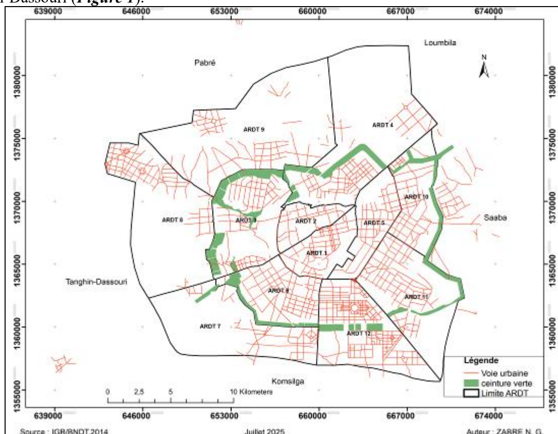
Figure 1. Présentation de la Zone d'étude (Source : IGB/BNDT, 2014).
