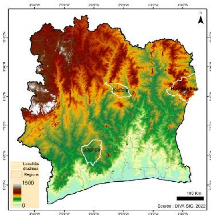
Figure 1. Situation géographique des départements d'étude
